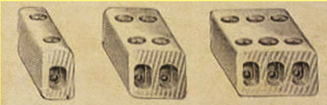
1925 Klammern: Eindraht, Zweidraht, Dreidraht ohne Montagebohrung (Petrier-Katalog, Ultimheat Museum)
